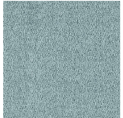
30/3272 blau-grün 93% Polyester, 7% Viskose Gewicht: 529g/m 2 Martindale: 100.000 Touren Lichtechtheit: 5 Pillingbildung: 4
