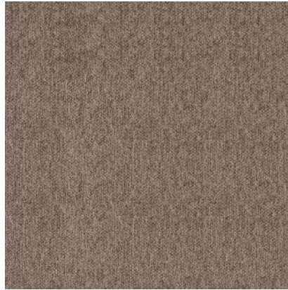
30/3268 dunkelbraun 93% Polyester, 7% Viskose Gewicht: 529g/m 2 Martindale: 100.000 Touren Lichtechtheit: 5 Pillingbildung: 4
