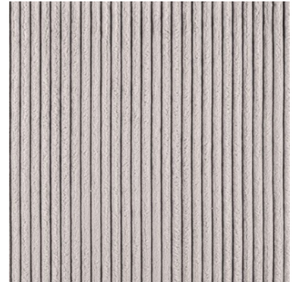
30/3278 hellgrau 92% Polyester, 8% Nylon Gewicht: 329g/m 2 Martindale: 100.000 Touren Lichtechtheit: 5 Pillingbildung: 4
